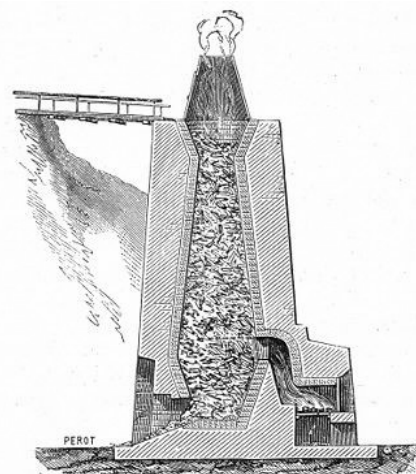
Fig. 78. — Four à chaux.
